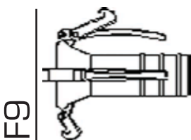
накрайник оребрен поцинкован женски с три куки female galvanized coupling with hose tail with three hooks
