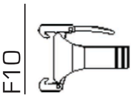
накрайник оребрен поцинкован женски female galvanized coupling with hose tail
